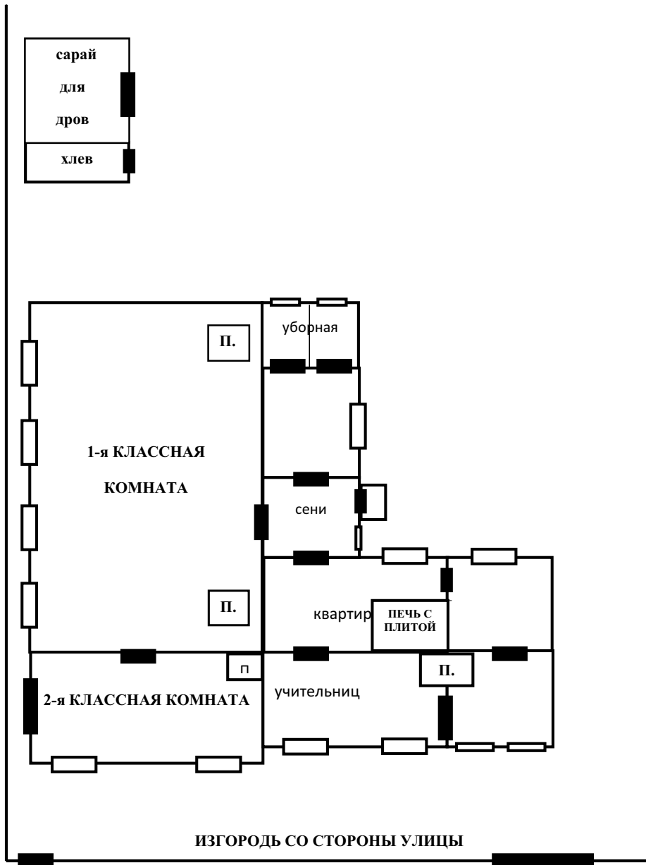
Прорисовка плана Нечепертской школьной усадьбы, 1921 г.
