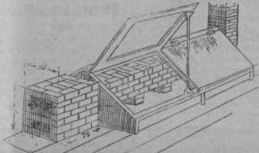
Печь Бурова № 200-300 Цыплят
