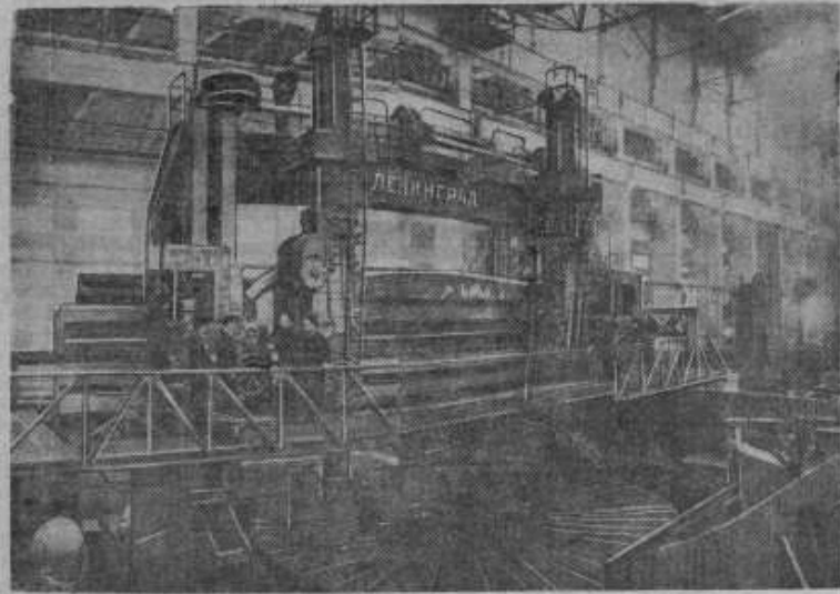
Завод имени Свердлова собрал и смонтировал в гидротурбинном цехе Металлического завода имени Сталина (Ленинград) наружный станок-гранулятор. Диаметр планшайбы станка — почти 9 метров. На нем можно обрабатывать детали до 170 тонн. Управление станком — автоматизированное — осуществляется с двух пультов. На снимке: общий вид нового наружного станка-гранулятора. Фото А. Михайлова (Фотохроника ТАСС.)
